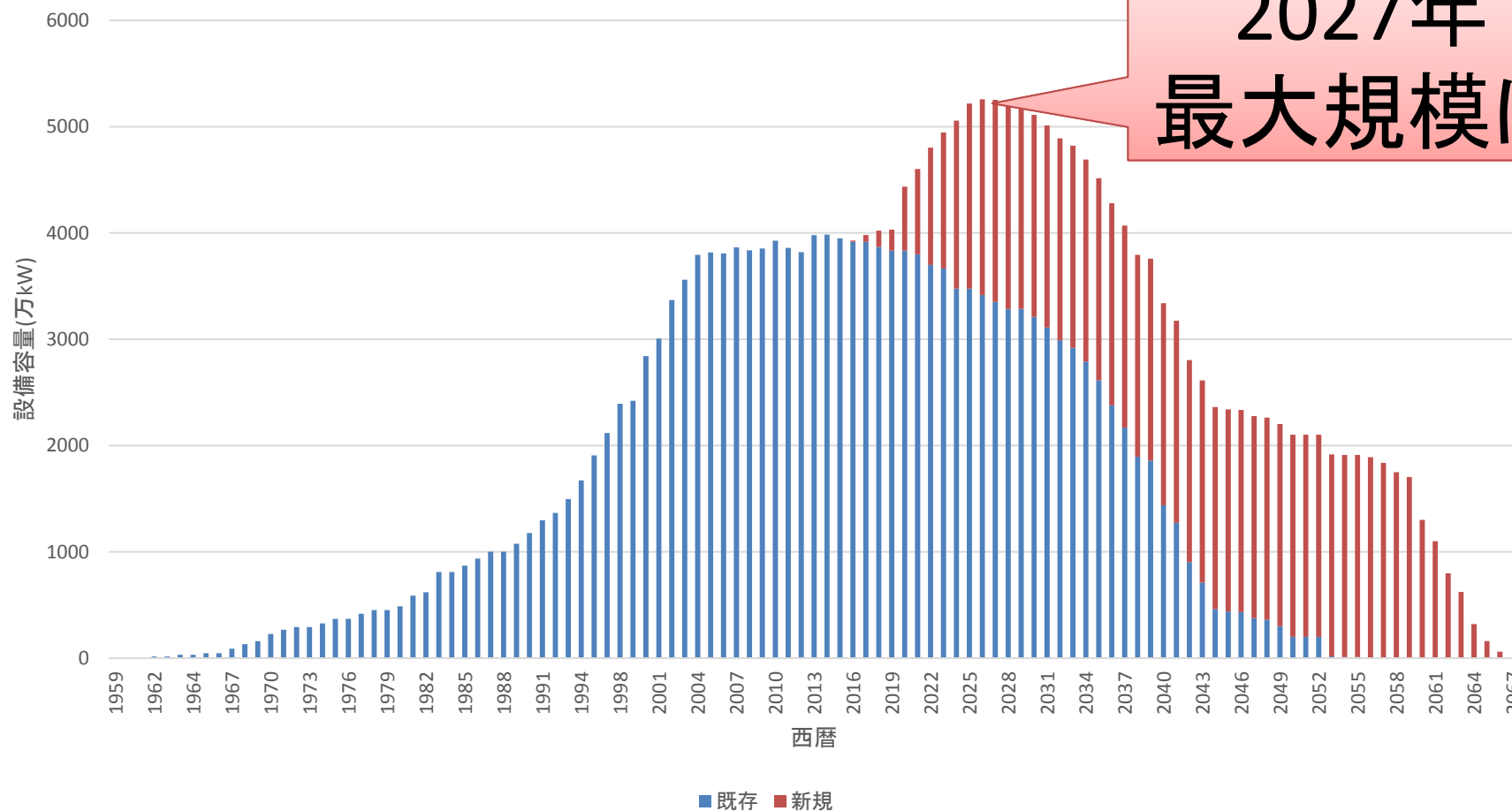
石炭火力発電所の設備容量累積(40年廃止)
